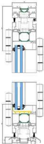
Coupe verticale
